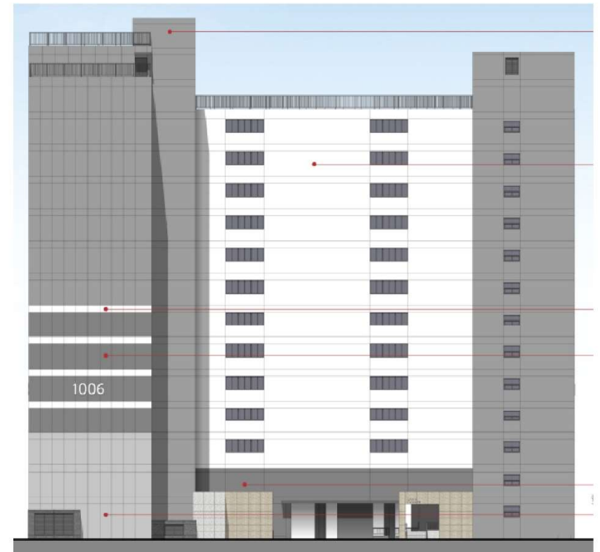
1006동(배면도)
